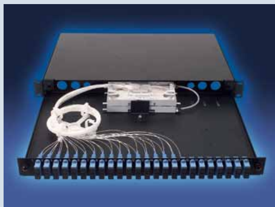
Полка со встроенными сплиттерами (высота 1U)
